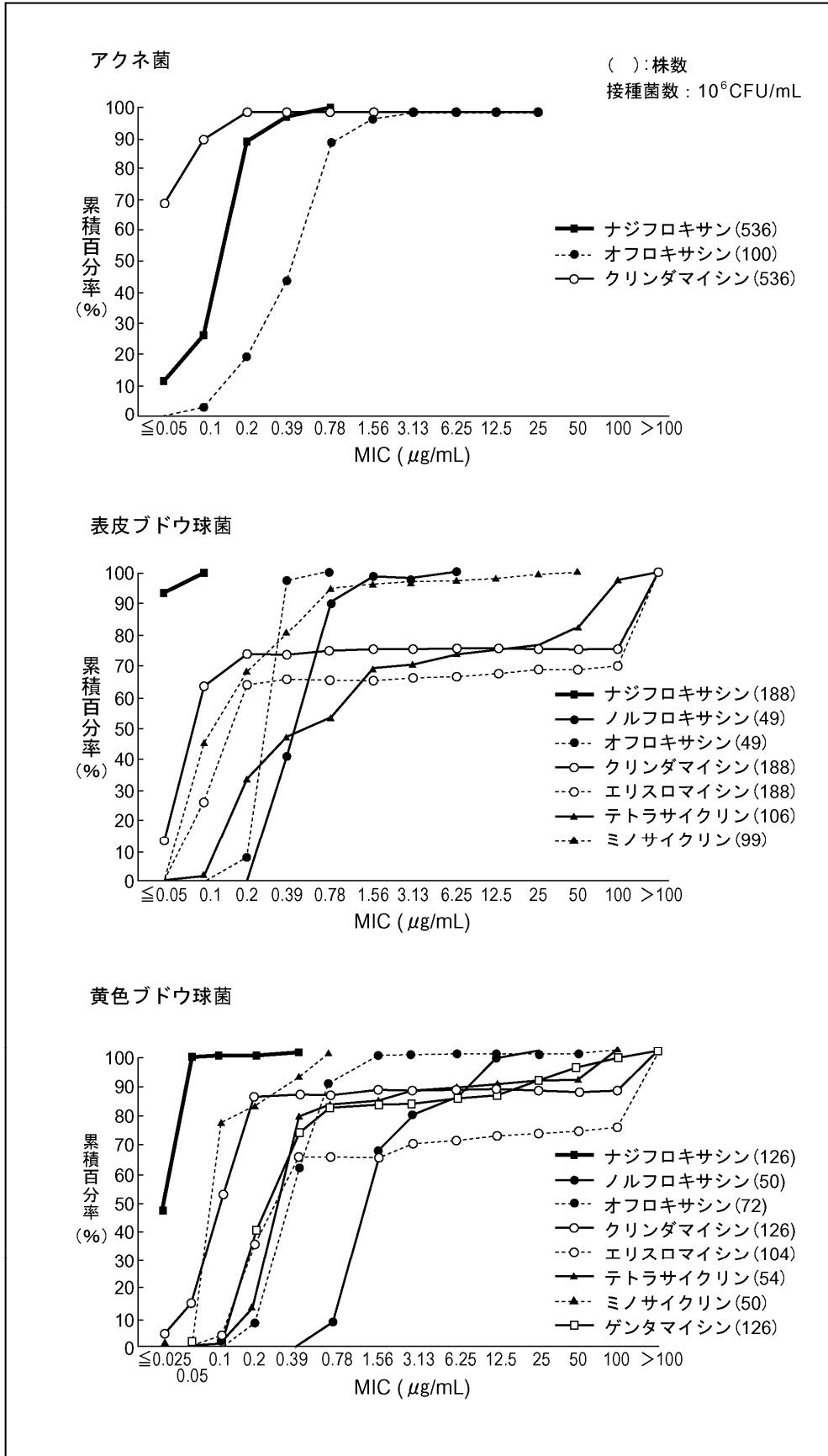
図3 臨床分離株に対する抗菌力
