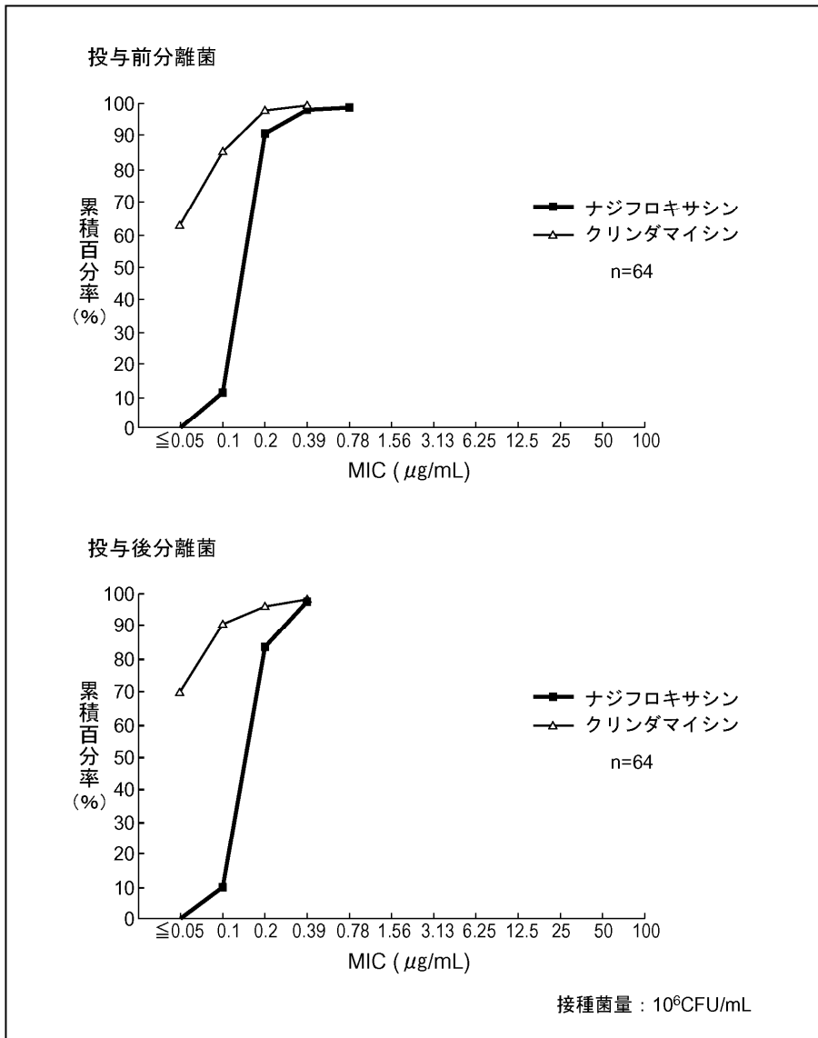
図5 ナジフロキサシン投与前後に同一ざ瘡*患者から分離されたアクネ菌に対する感受性
