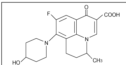
図1 ナジフロキサシンの構造式
