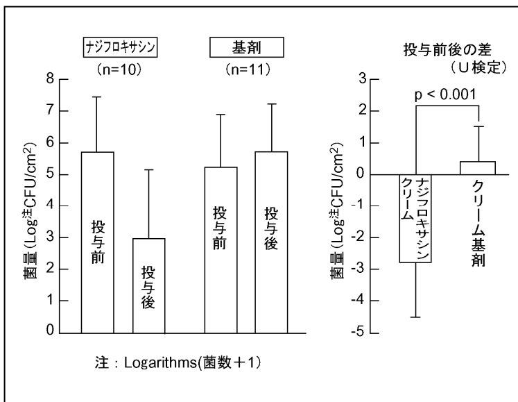
図8 ナジフロキサシンクリーム投与前後のアクネ菌の菌量変化
