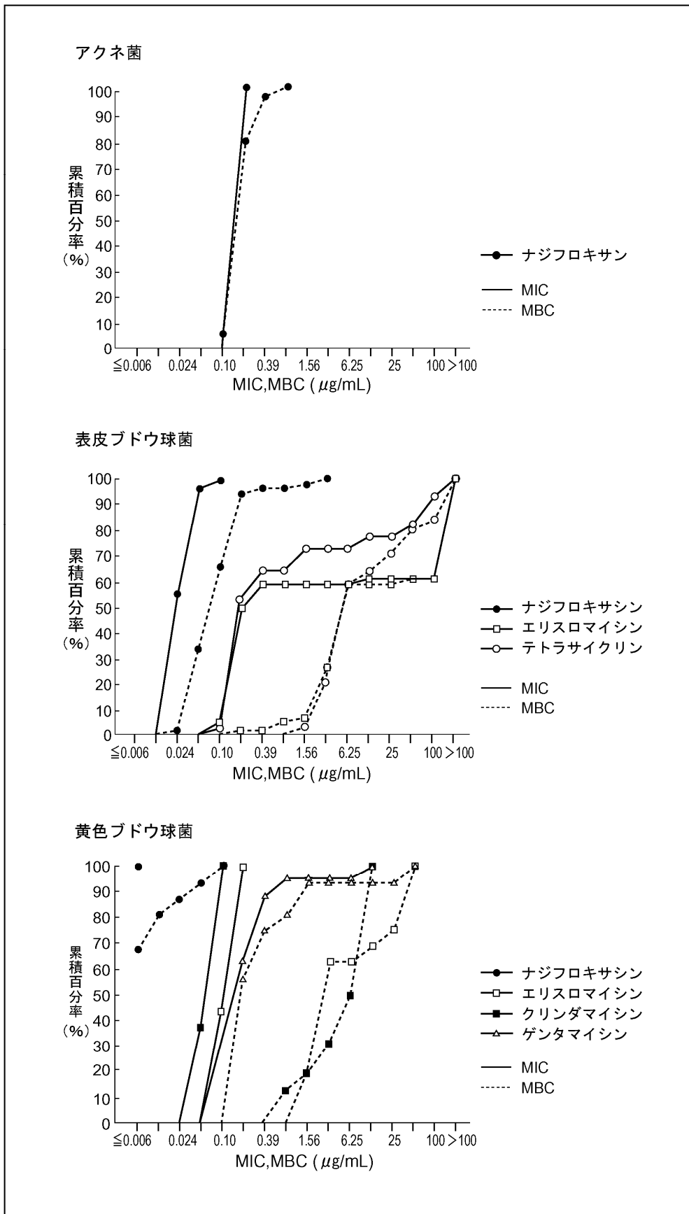
図 4 臨床分離株に対する MIC 及び MBC
