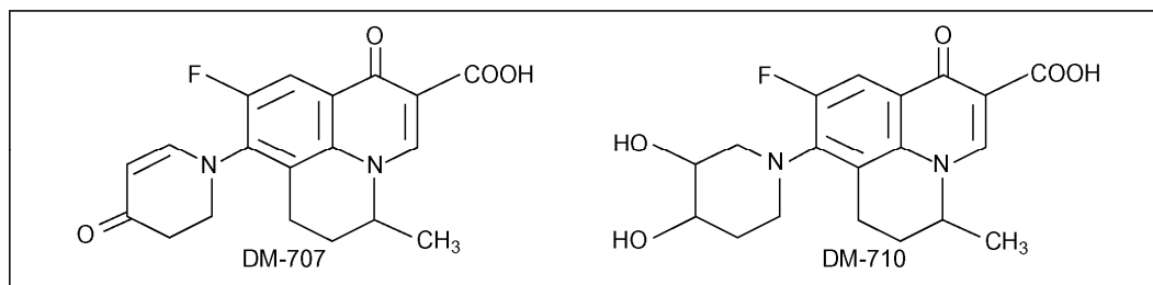
図9 ナジフロキサシンの代謝物（各種動物）
