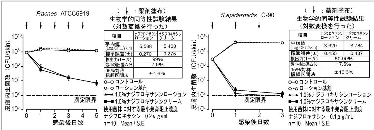
図7 ナジフロキサシン軟膏 1%の in vivoにおける抗菌活性
