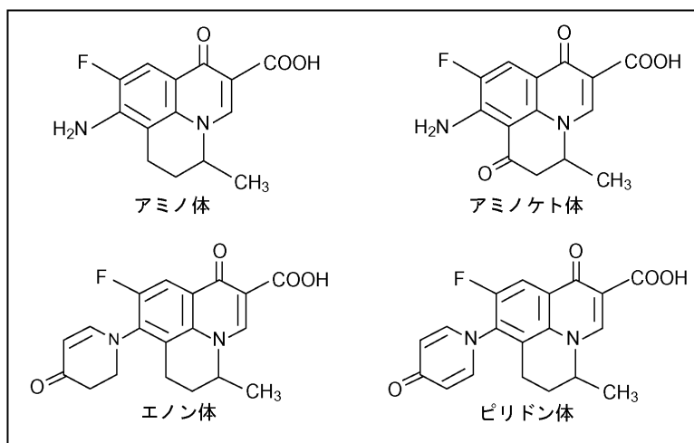
図2 ナジフロキサシンの強制分解による生成物
