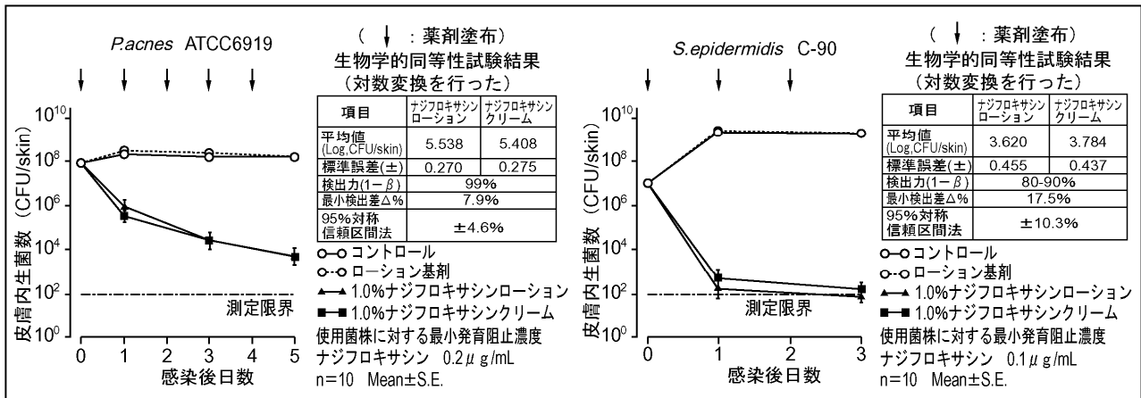
図 6 ナジフロキサシンローションの in vivo における抗菌活性
